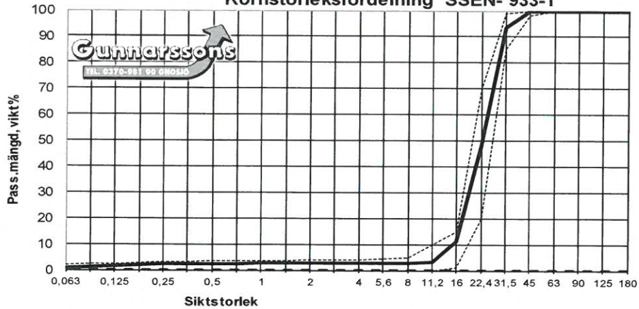
Kornstorleksfördelning SSEN- 933-1
